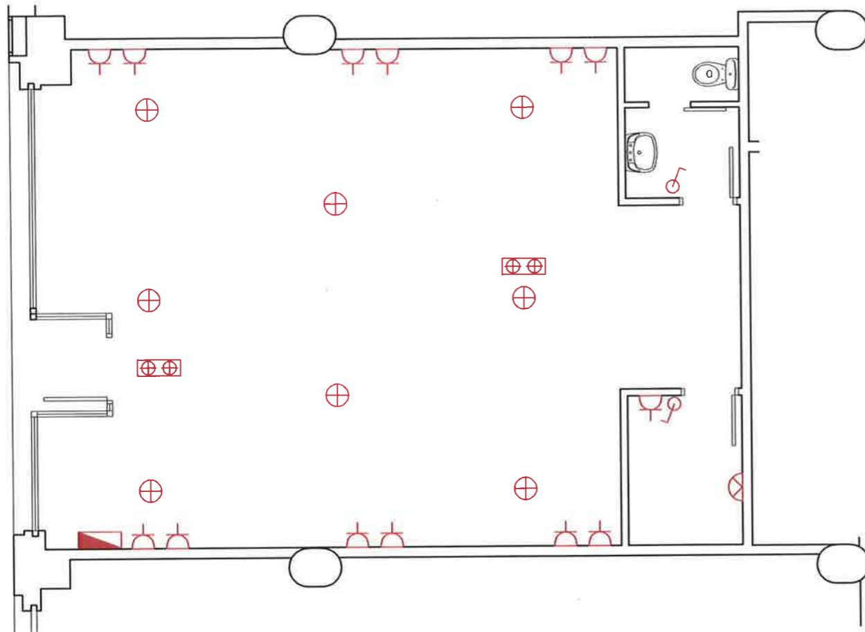
Planta local 6
